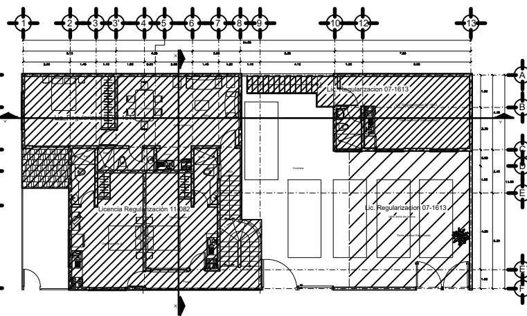
PLANTA PRIMER NIVEL
